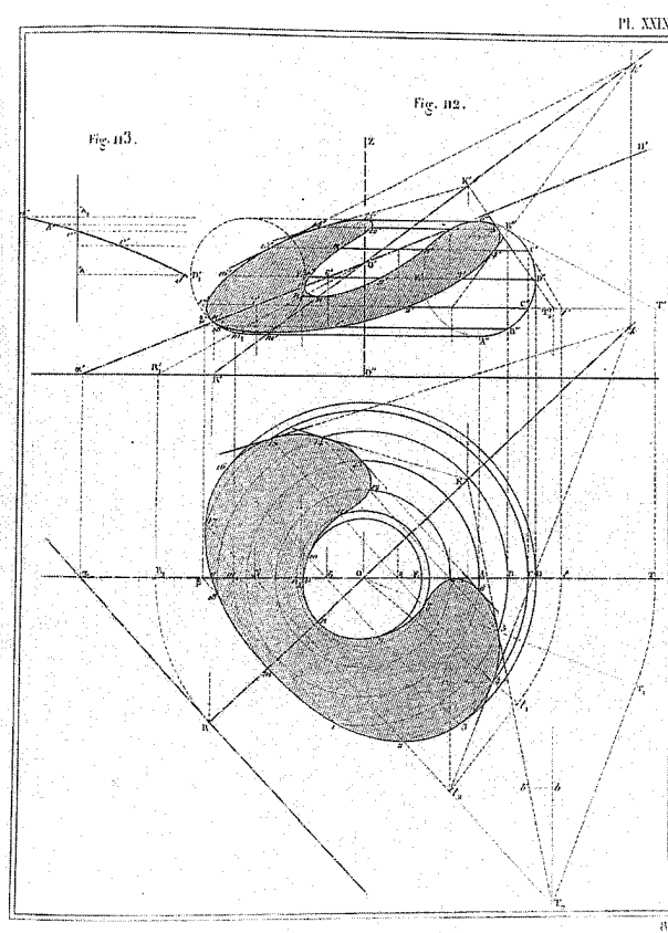
Epure tirée du Traité de géométrie descriptive de J. de La Gournerie. Intersection plane d'un surface de révolution (tome 1, 1873, pl. XXIX).
