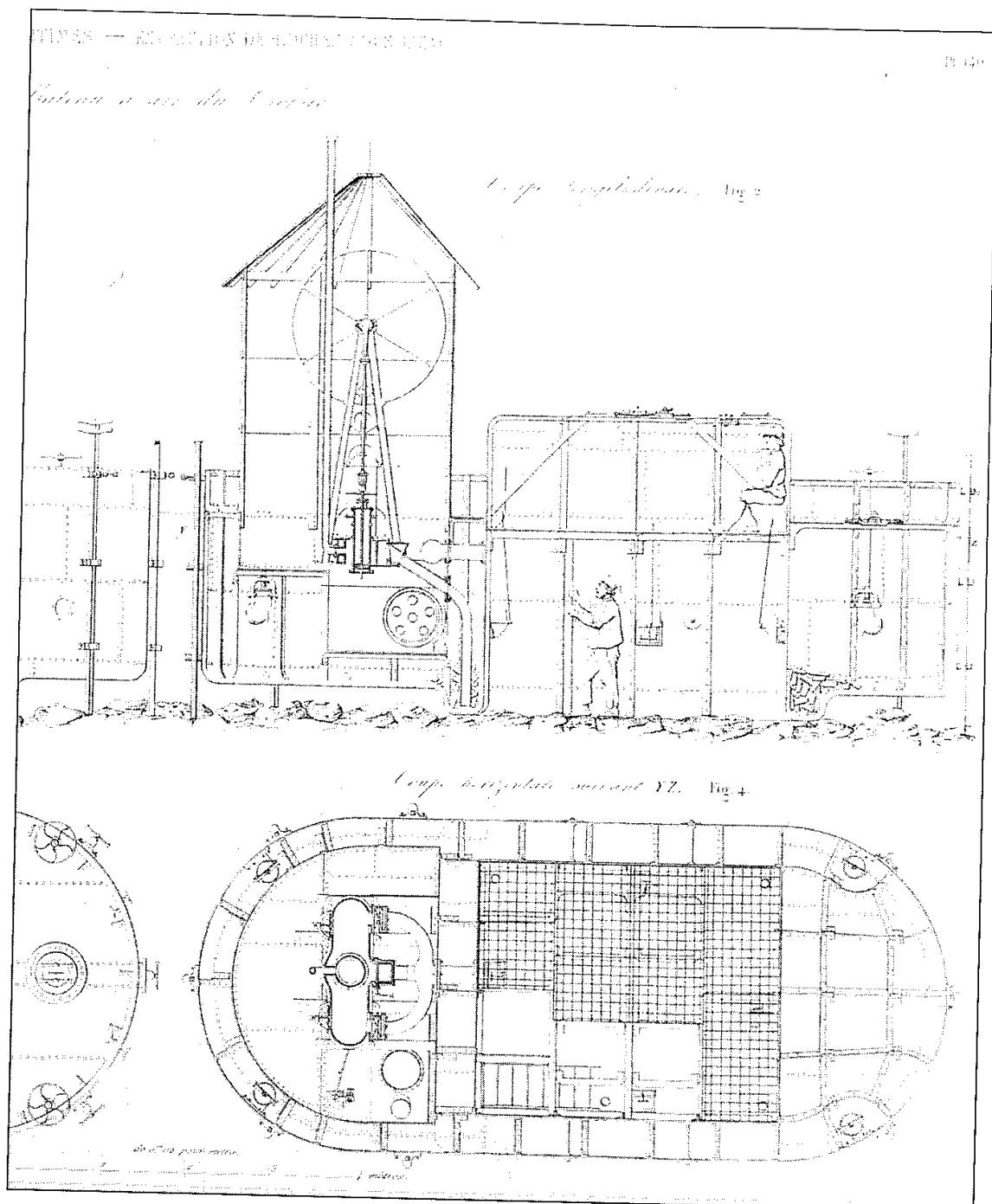
Deux coupes (longitudinale et horizontale) du bateau à air construit en 1846 par La Gournerie pour l'extraction de roches dans la passe du Croisic.
