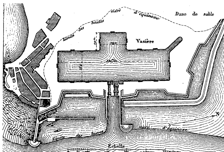
Projet de bassin à flot de Saint-Nazaire (plan de Jégou et La Gournerie) tel qu'il fut approuvé en 1847.
